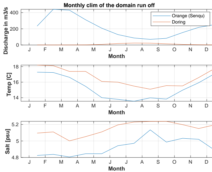
Figura 6: Serie de tiempo del caudal, temperatura y salinidad de los ríos disponible en el dominio. Figura emitada al finalizar de ejecutar make_runoff.
