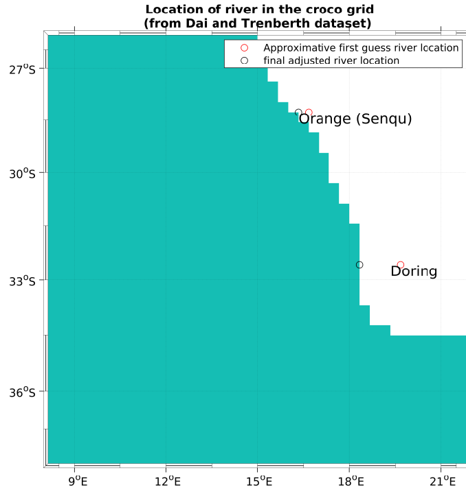
Figura 5: Ubicación de los ríos disponible en el dominio. Figura emitada al finalizar de ejecutar make_runoff.
