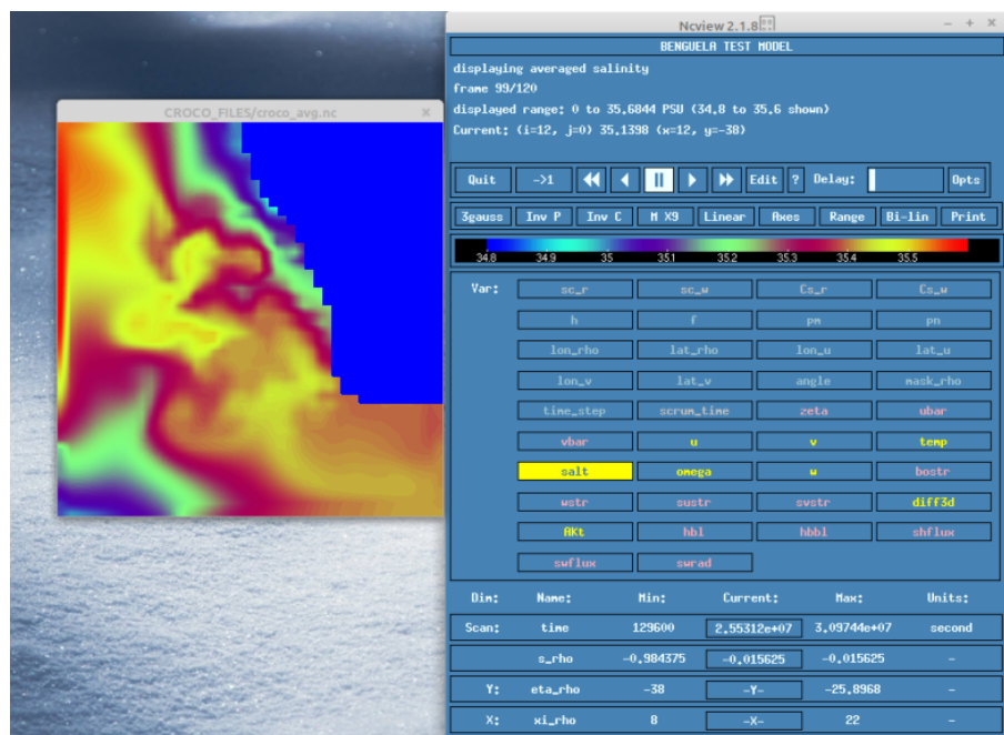
Figura A4: Caso 2b: Salinidad superficial en t=28 obtenido de croco_avg.nc (rango 34.6-35.6 psu)
