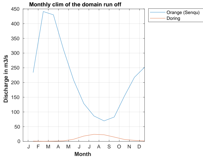
Figura 4: Serie de tiempo del caudal de los ríos disponible en el dominio. Figura emitada durante make_runoff.
