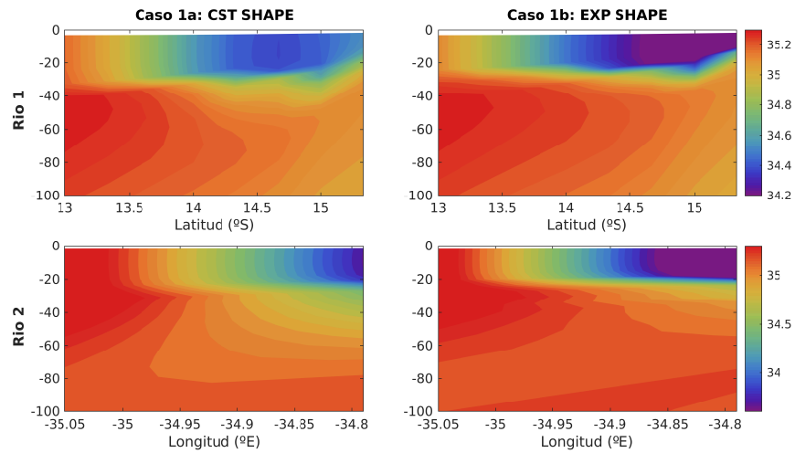
Figura A3: Secciones verticales de la salinidad, perpendicular a la boca de Rio 1 (arriba) y 2 (abajo). Izquierda (Derecha), Sección utilizando configuración CST_SHAPE (EXP_SHAPE)
