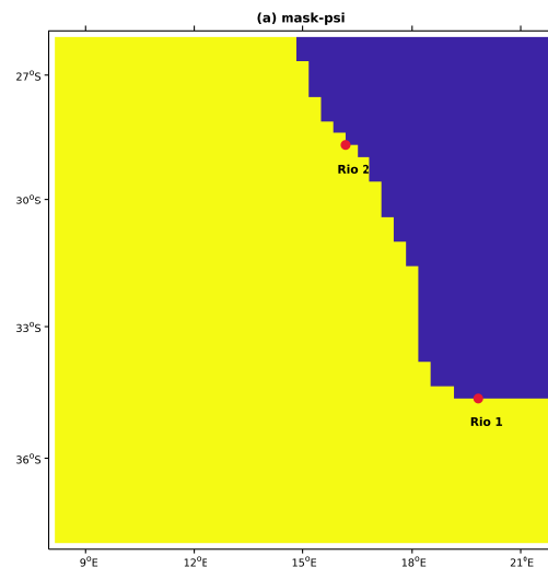
Figura 1: Posición de los ríos para el Caso 1a.
