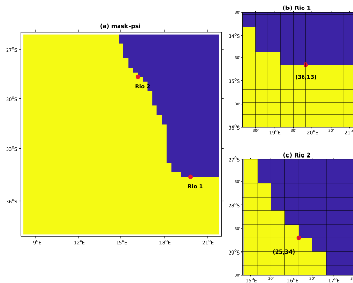
Figura A1: (a) Máscara en coordenadas psi donde se muestra la posición de los ríos 1 y 2. (b) y (c) Zoom de Río 1 y 2, respectivamente
