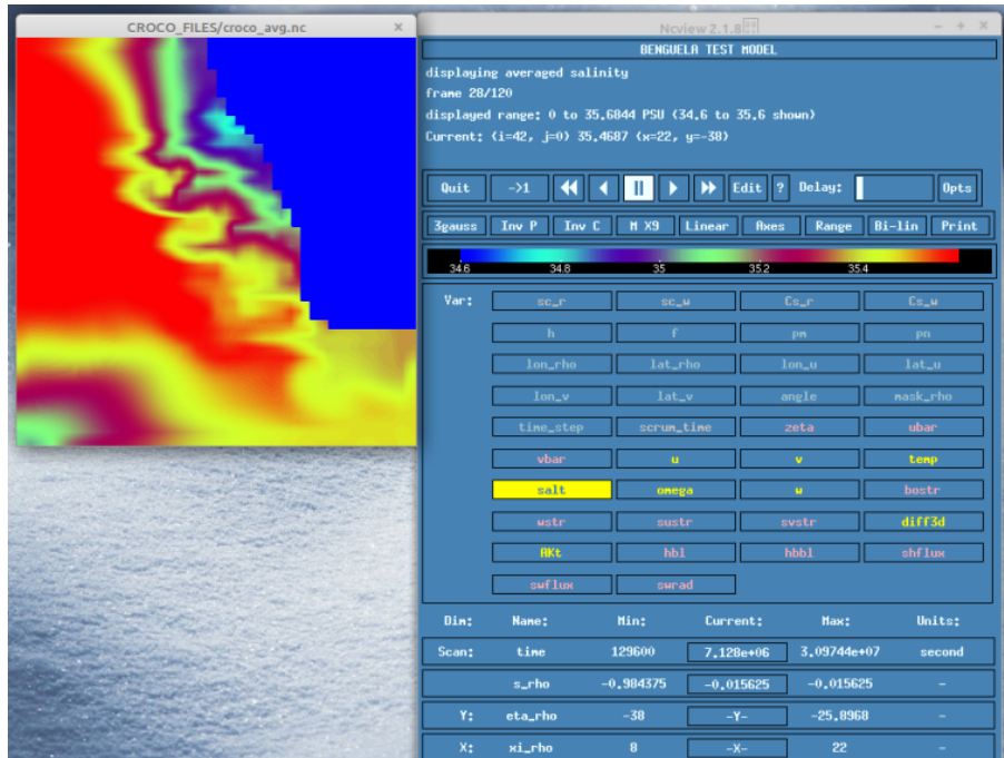
Figura 7: Caso 2a: Salinidad superficial en t=28 obtenido de croco_avg.nc (rango 34.6-35.6 psu)
