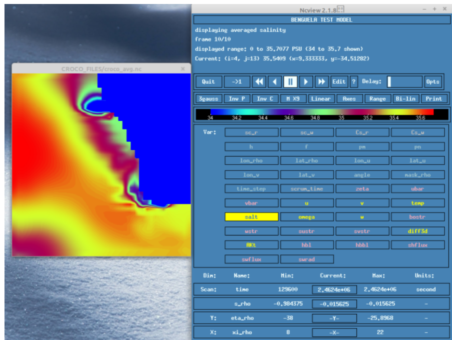
Figura A2: Caso 1b: Salinidad superficial en t=10 , obtenido de croco_avg.nc (rango 34-35.7 psu)
