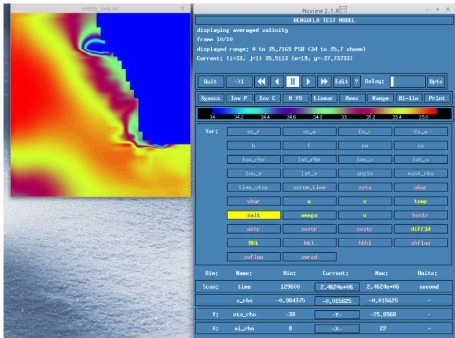
Figura 2: Caso 1a: Salinidad superficial en t=10 obtenido de croco_avg.nc (rango 34-35.7 psu)
