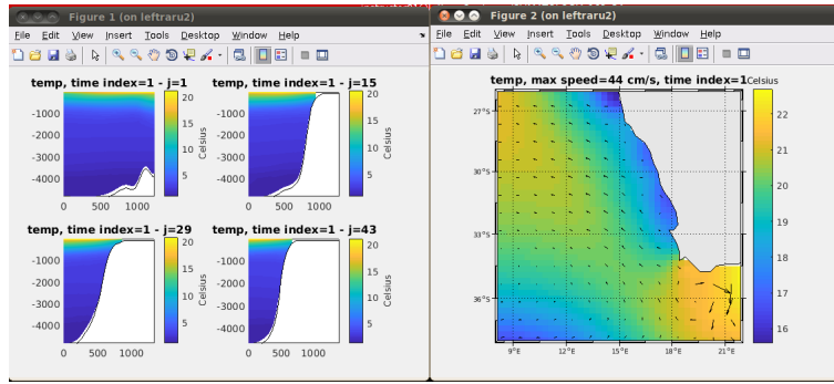
Figura 7: Variables de forzamiento lateral oceánico: temperatura en secciones verticales y en superficie en t = 1 .
