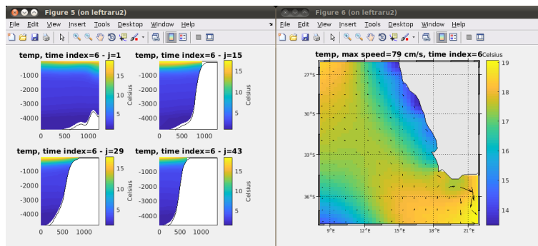
Figura 9: Variables de forzamiento lateral oceánico: temperatura en secciones verticales y en superficie en t = 6 .
