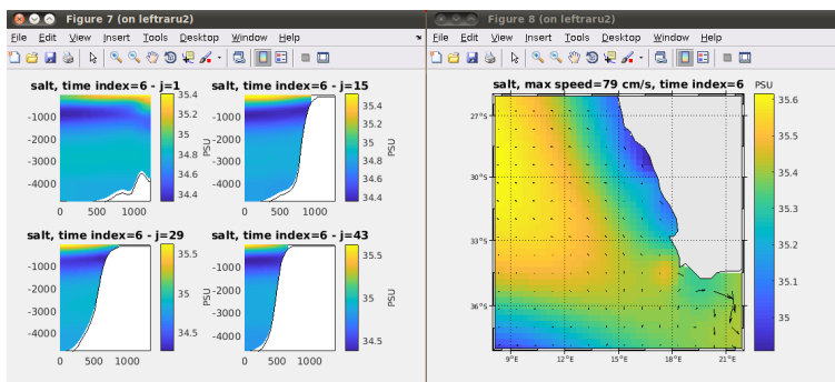
Figura 10: Variables de forzamiento lateral oceánico: salinidad en secciones verticales y en superficie en t = 6 .
